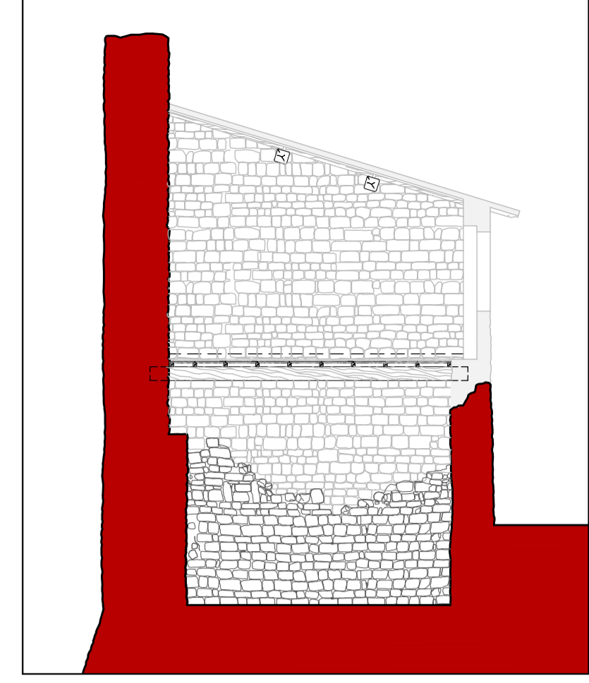
SEZIONE A-A SCALA 1:100
