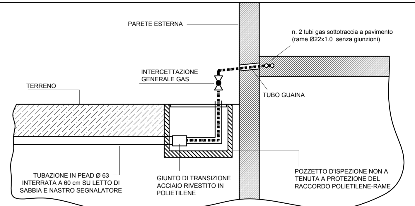
TUBAZIONE GAS GPL PARTICOLARE POZZETTO
