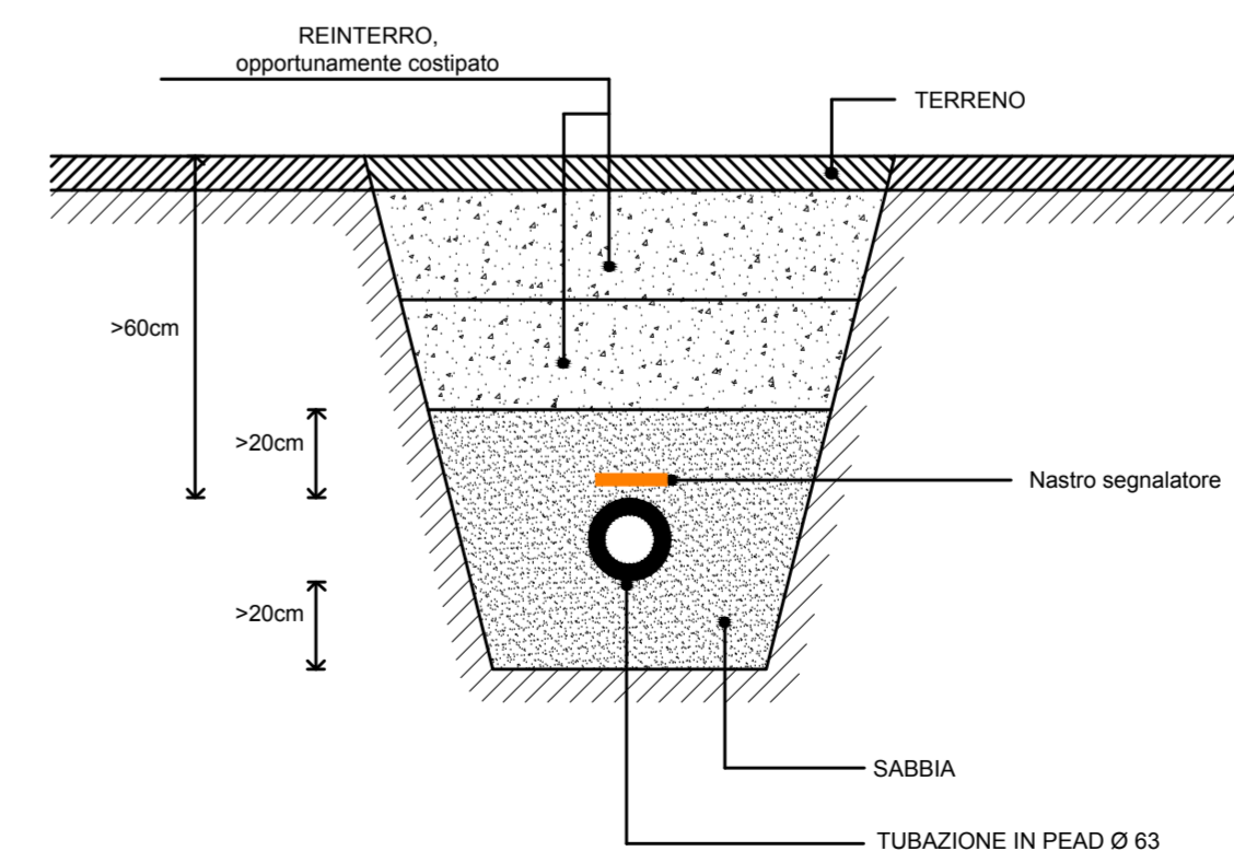
TUBAZIONE GAS GPL PARTICOLARE SCAVO
