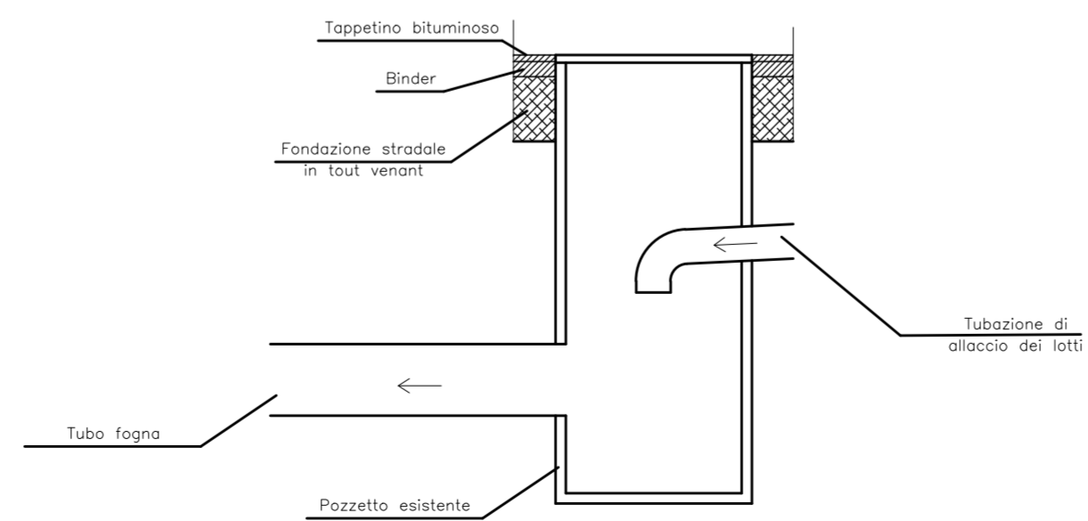
PARTICOLARE RECAPITO ACQUE NERE AL POZZETTO DELLA FOGNATURA PUBBLICA ESISTENTE
