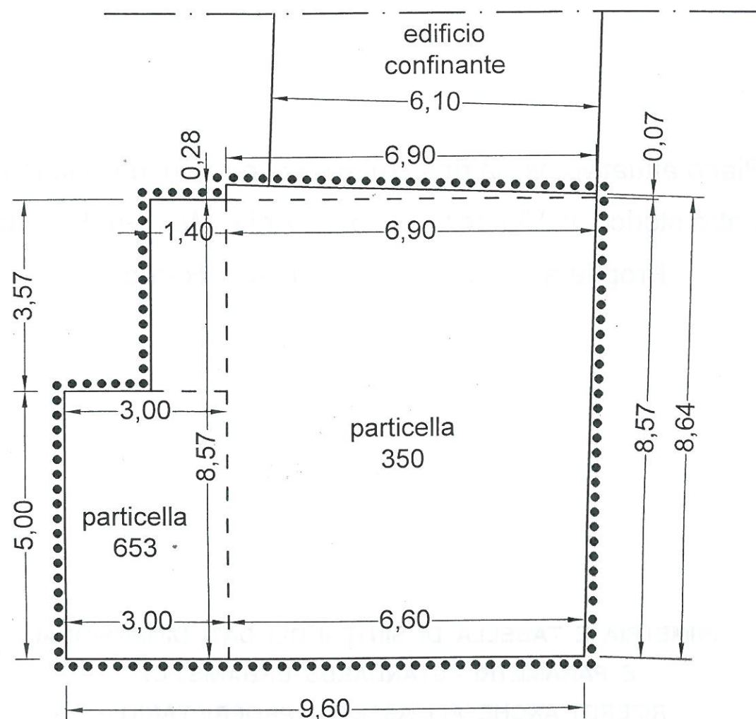
PLANIMETRIA DEL PIANO TERRA
