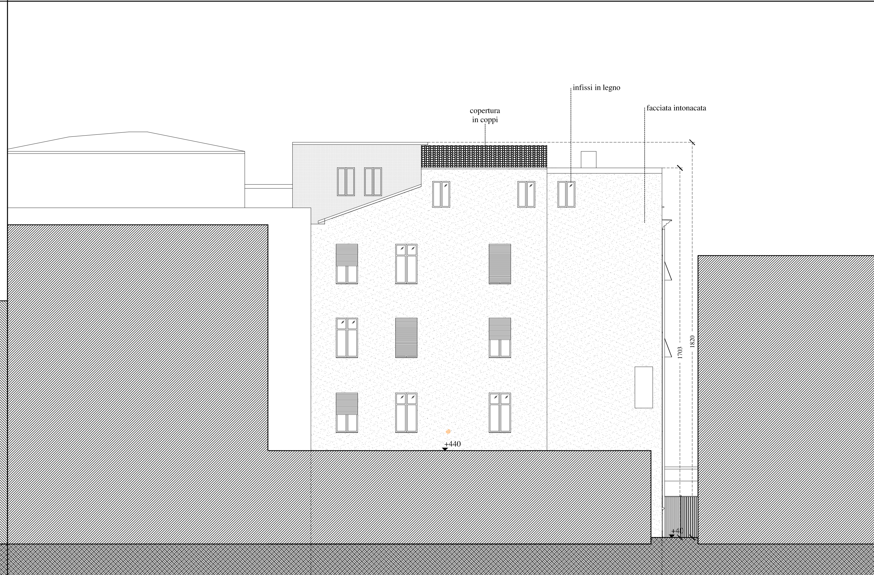
----- 1618 ----- EDIFICIO OGGETTO DI INTERVENTO
