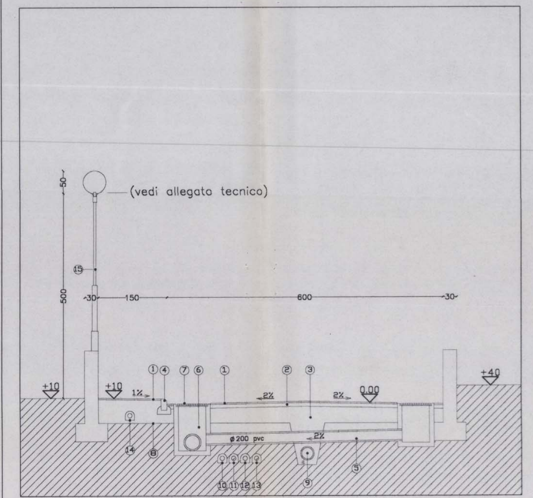
Sezione stradale tipo scala 1:50
