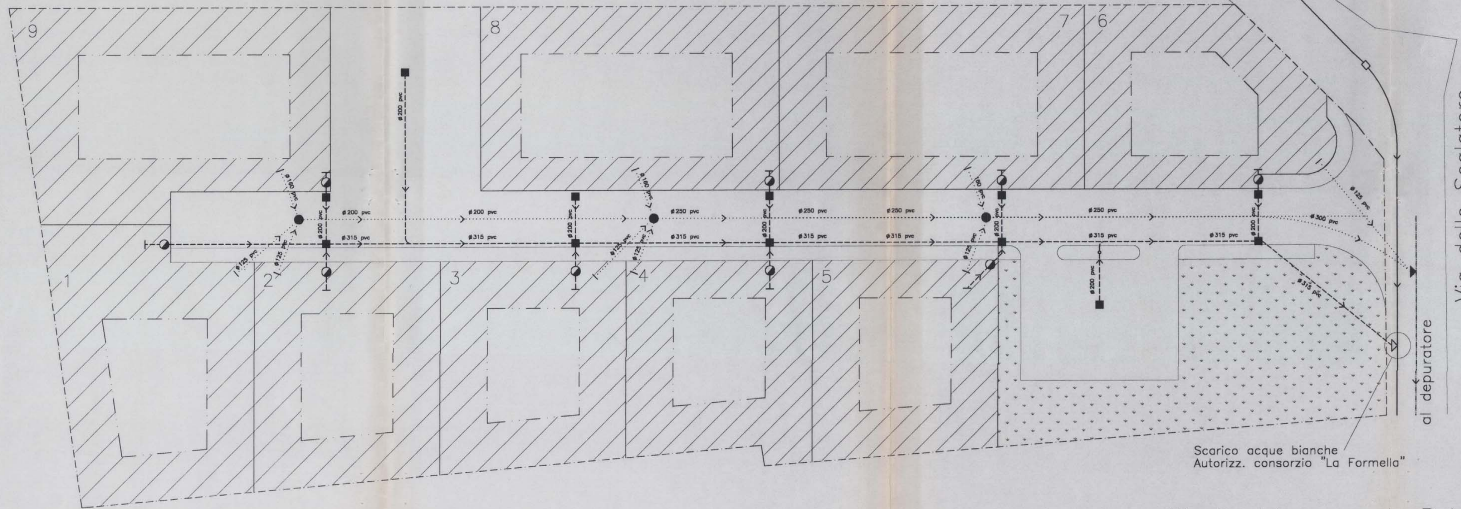
Planimetria generale Rete fognante scala 1:250
