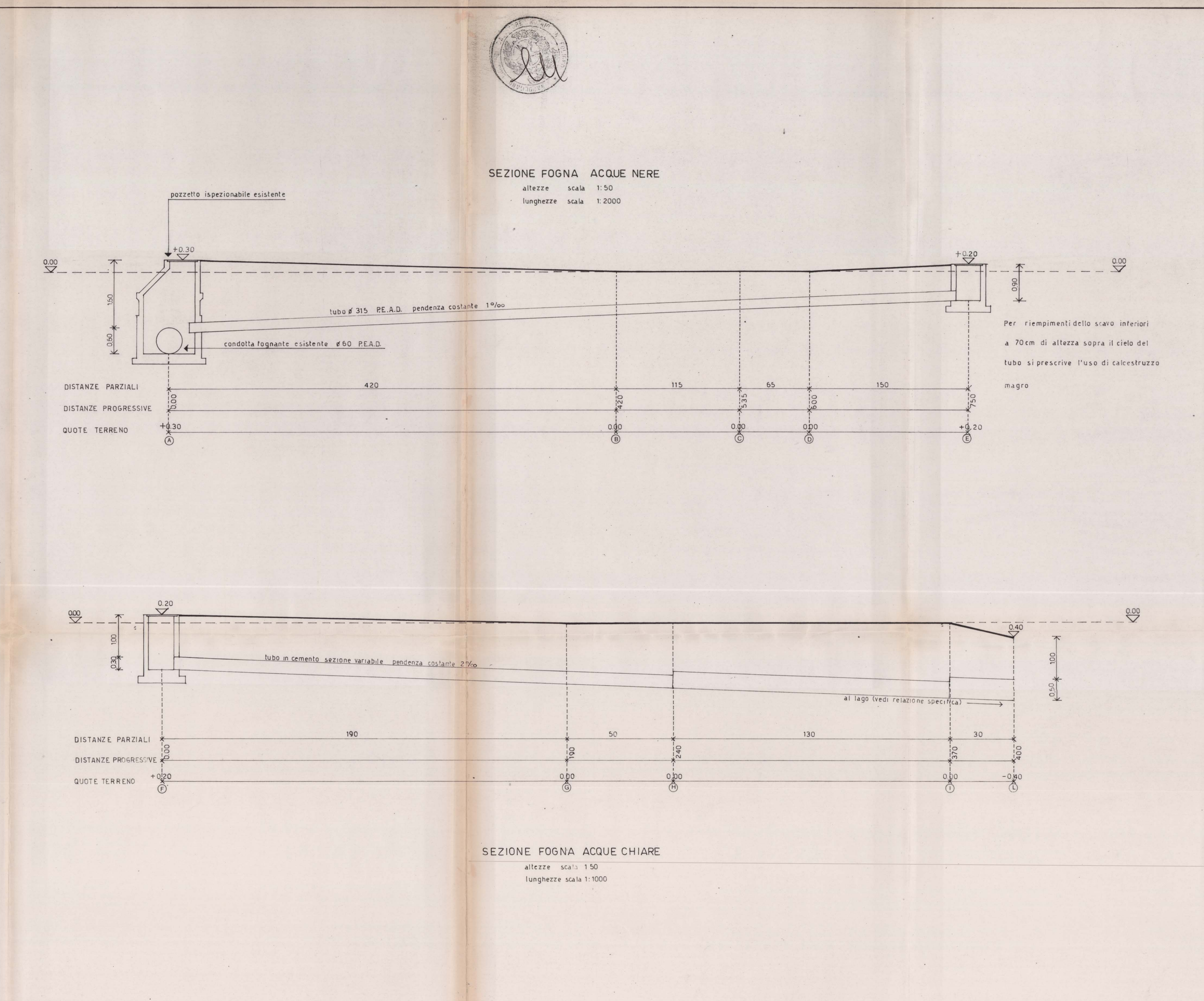
PARTICOLARI DELLA FOGNATURA PUBBLICA
