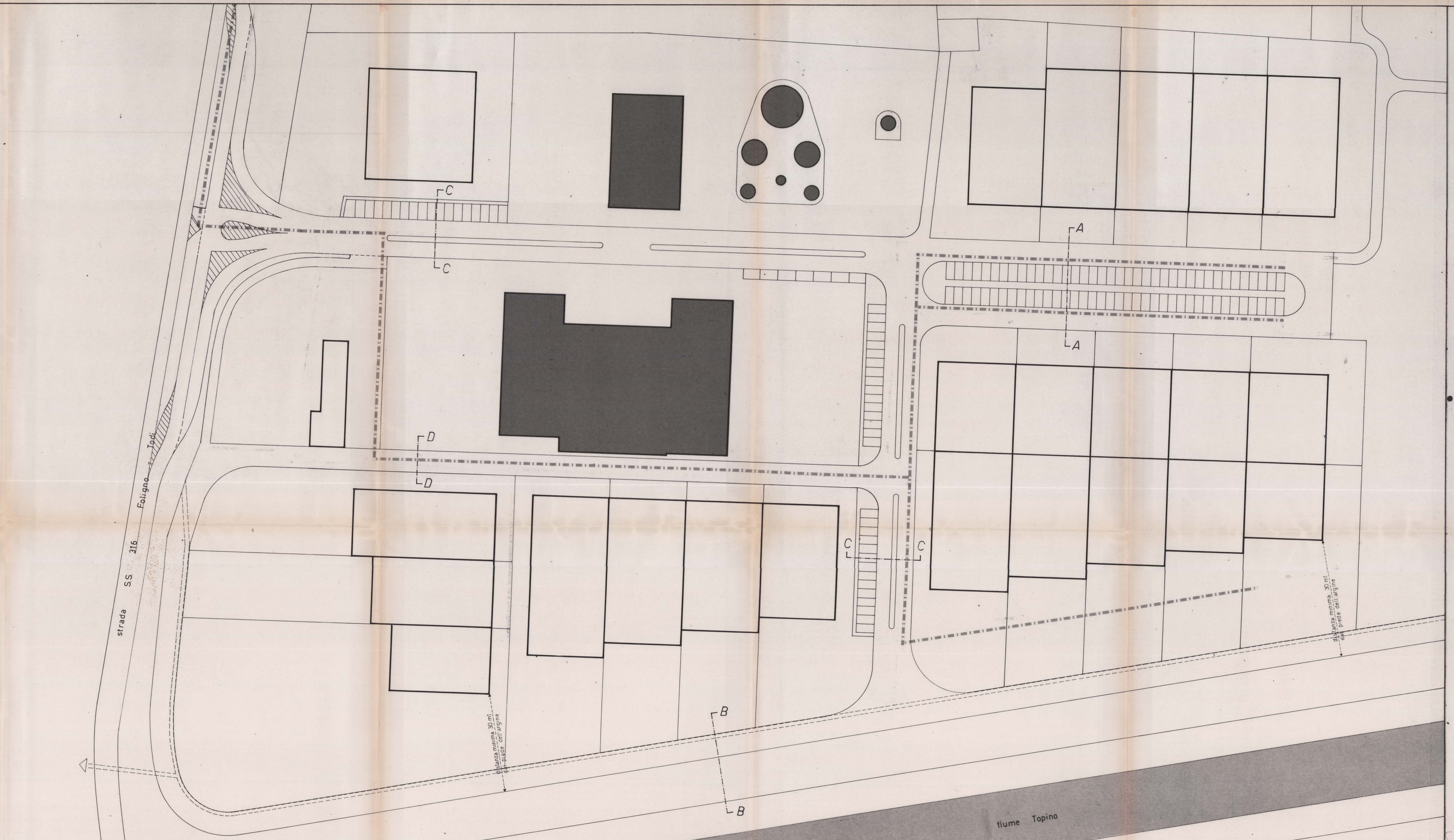
SCHEMA GENERALE RETE IDRICA E GAS scala 1:2000
