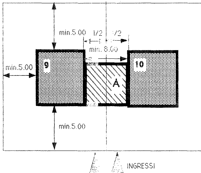
Schema di pianta mc 2100+2100
