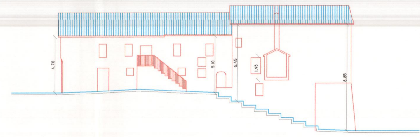
PROFILO P-P
