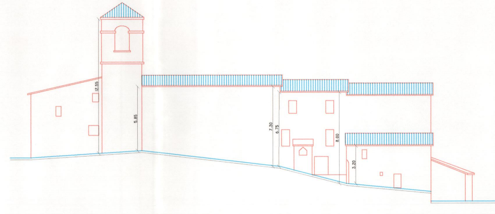
PROFILO R-R
