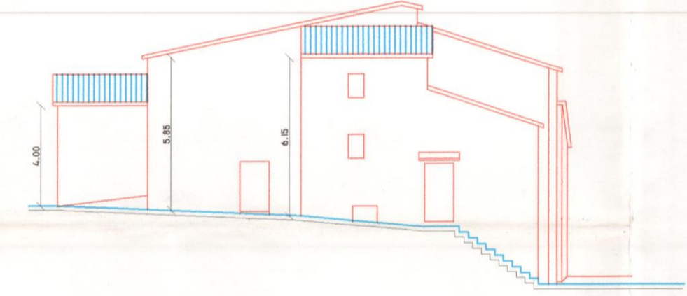
PROFILO T-T
