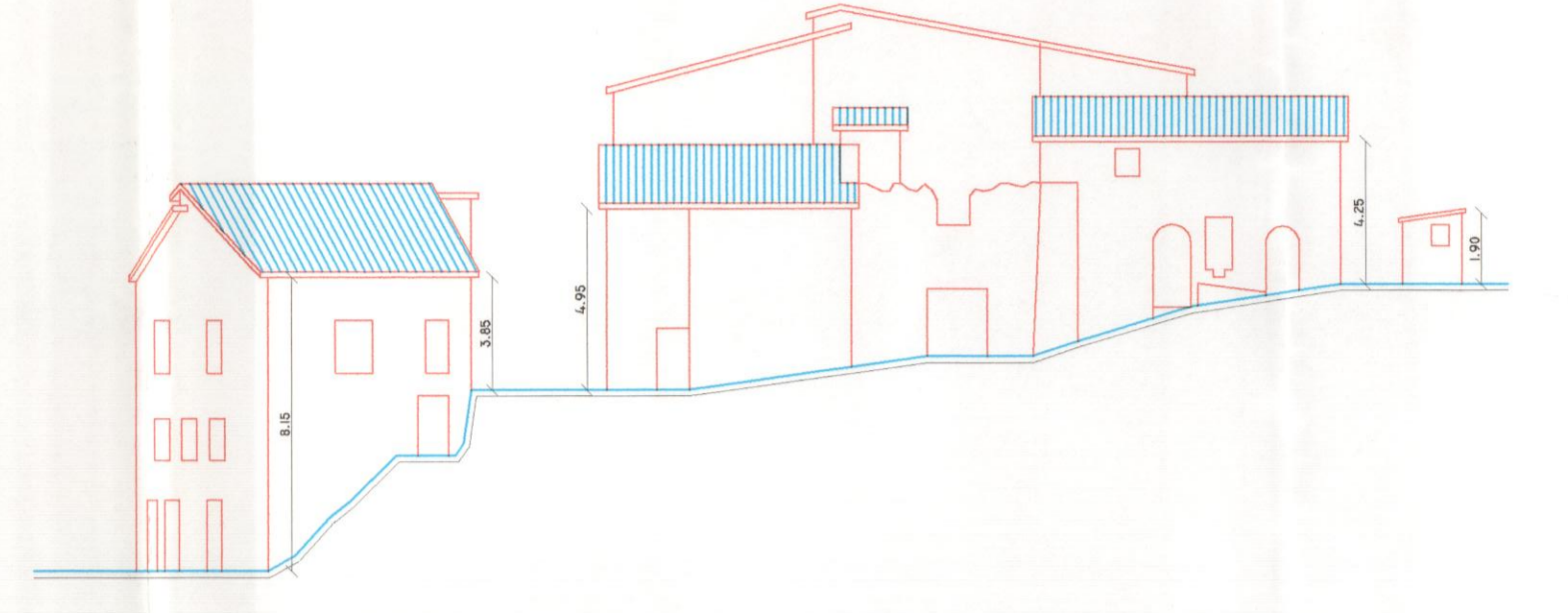
PROFILO S-S
