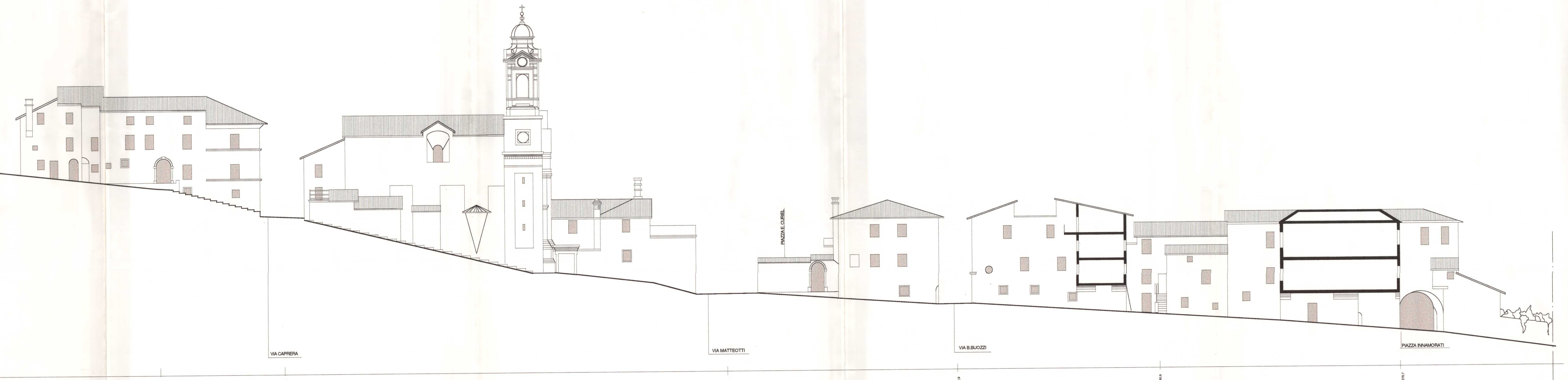
PROSPETTO B-B
