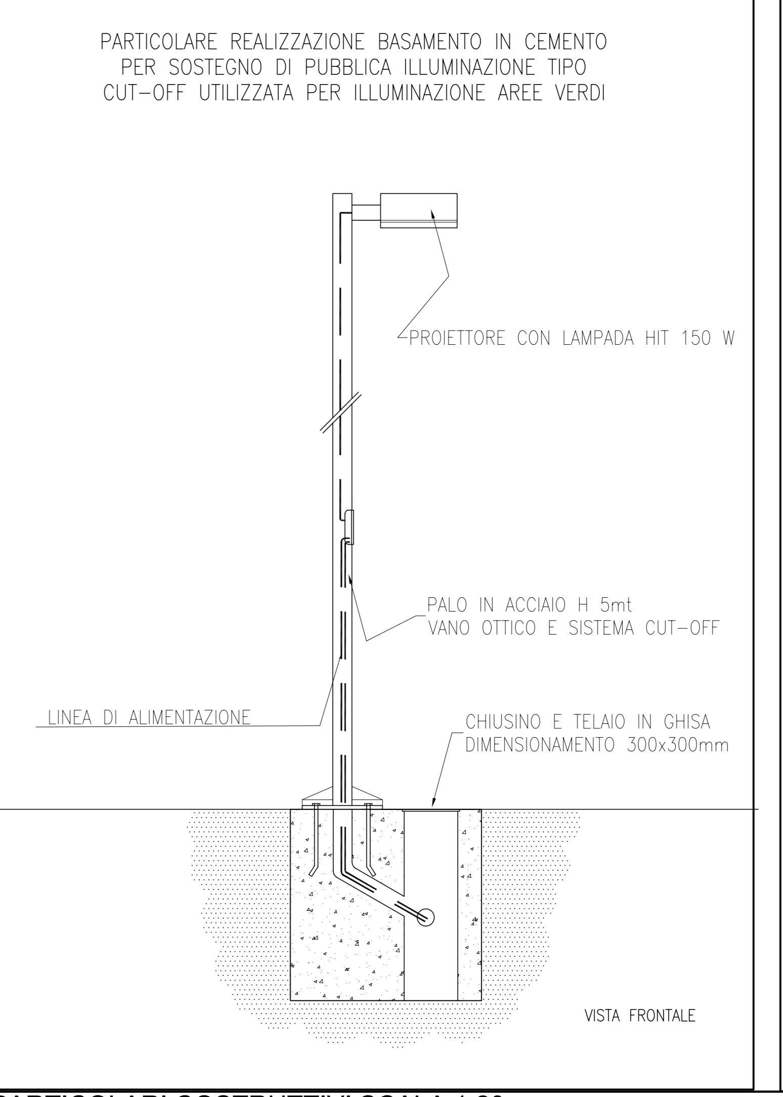
PARTICOLARI COSTRUTTIVI SCALA 1:20
