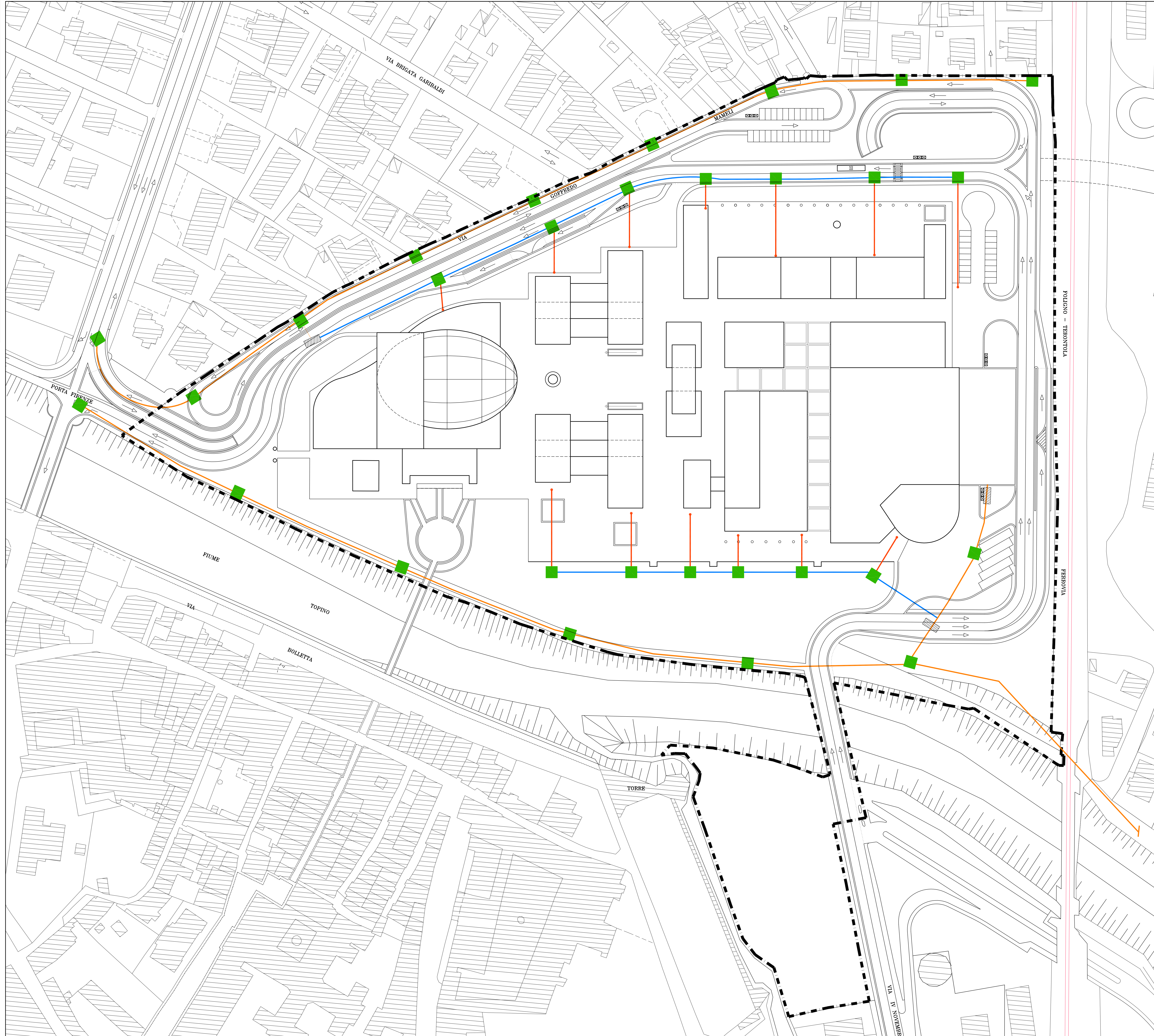
PLANIMETRIA SCALA 1:500
